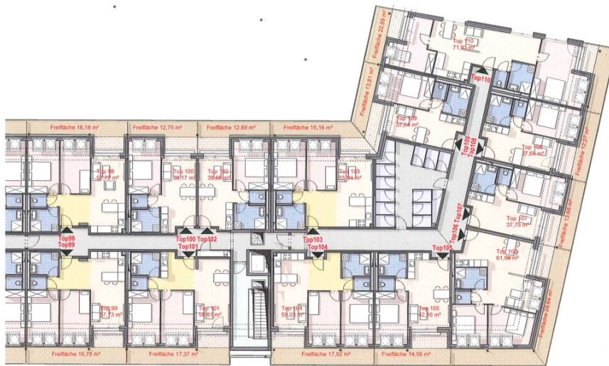
GESAMTPLAN 1.DG B
