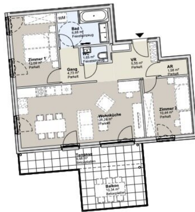
1. DACHGESCHOSS GARTENBAUKÖRPER
