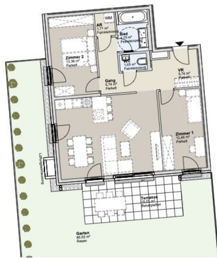
ERDGESCHOSS GARTENBAUKÖRPER
