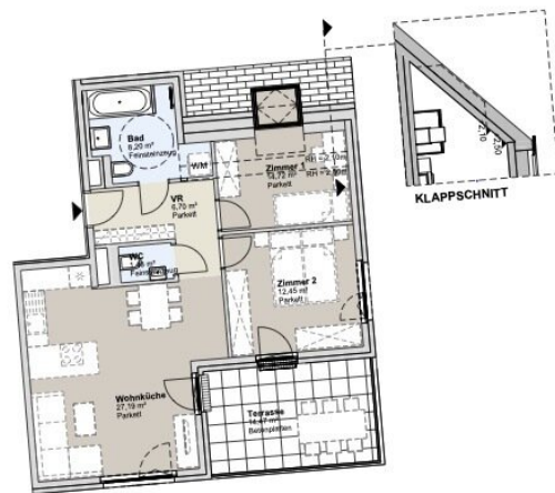
2. DACHGESCHOSS GARTENBAUKÖRPER
