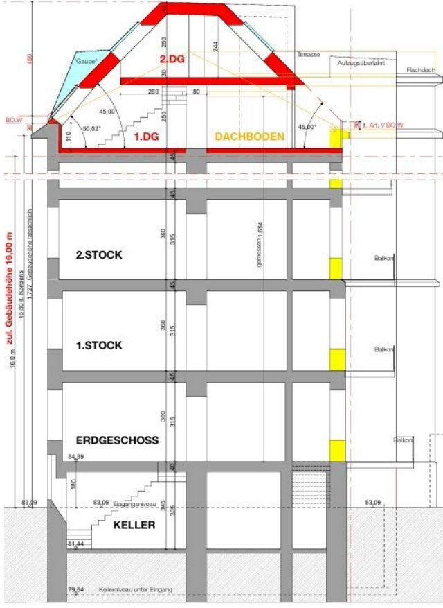
VORENTWURF
