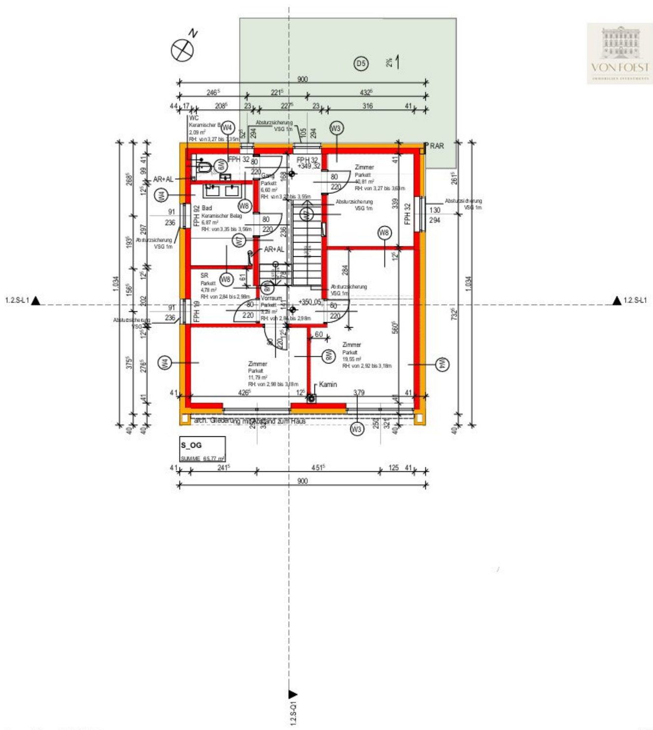
Grundriss 1.2.S-OG
