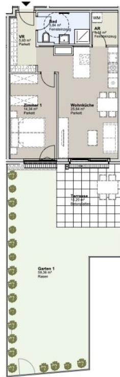
ERDGESCHOSS STRASSENBAUKÖRPER
