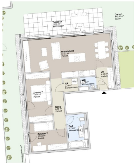
ERDGESCHOSS GARTENBAUKÖRPER
