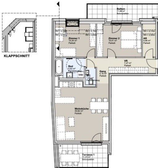
1. DACHGESCHOSS STRASSENBAUKÖRPER
