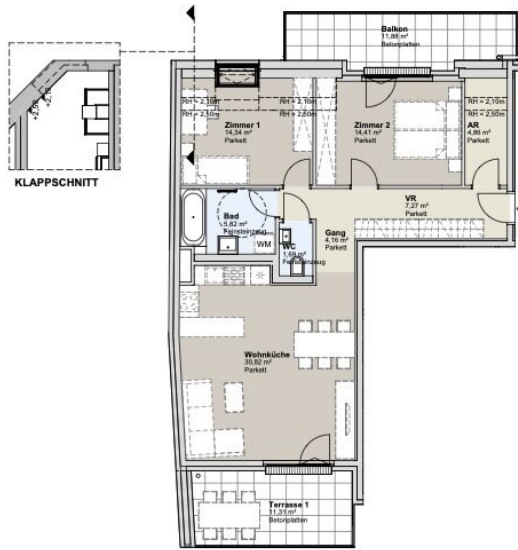
1. DACHGESCHOSS STRASSENBAUKÖRPER
