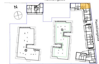
ÜBERSICHTSPLAN- 3.OG
