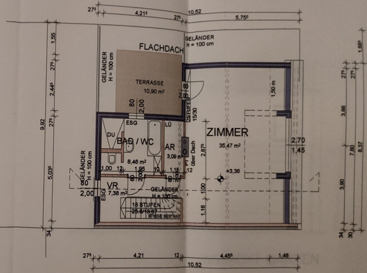
GRUNDRISS DG
