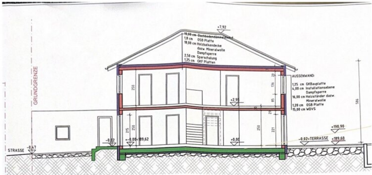
SCHNITT A-A
