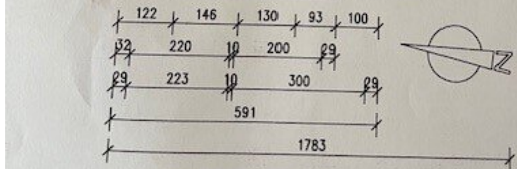
GRUNDRISS DG M 1:100 NUTZFLÄCHE DG = 41,85 M 2
