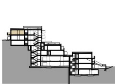
SCHNITT BK 02+04
