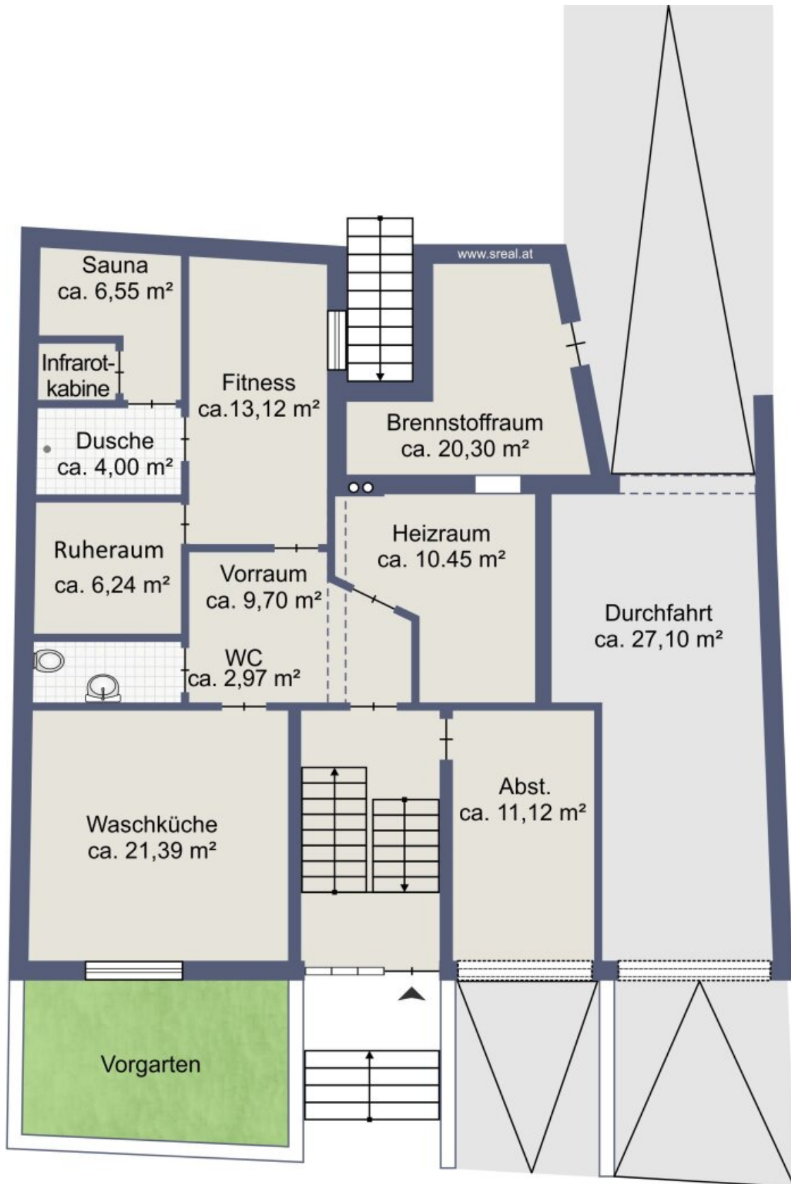
Skizze Kellergeschoss
