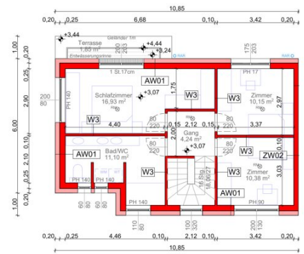
GRUNDRISS OBERGESCHOSS 1:100
