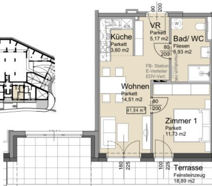
GRUNDRISS BK 01
