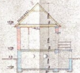
SCHNITT A-B
