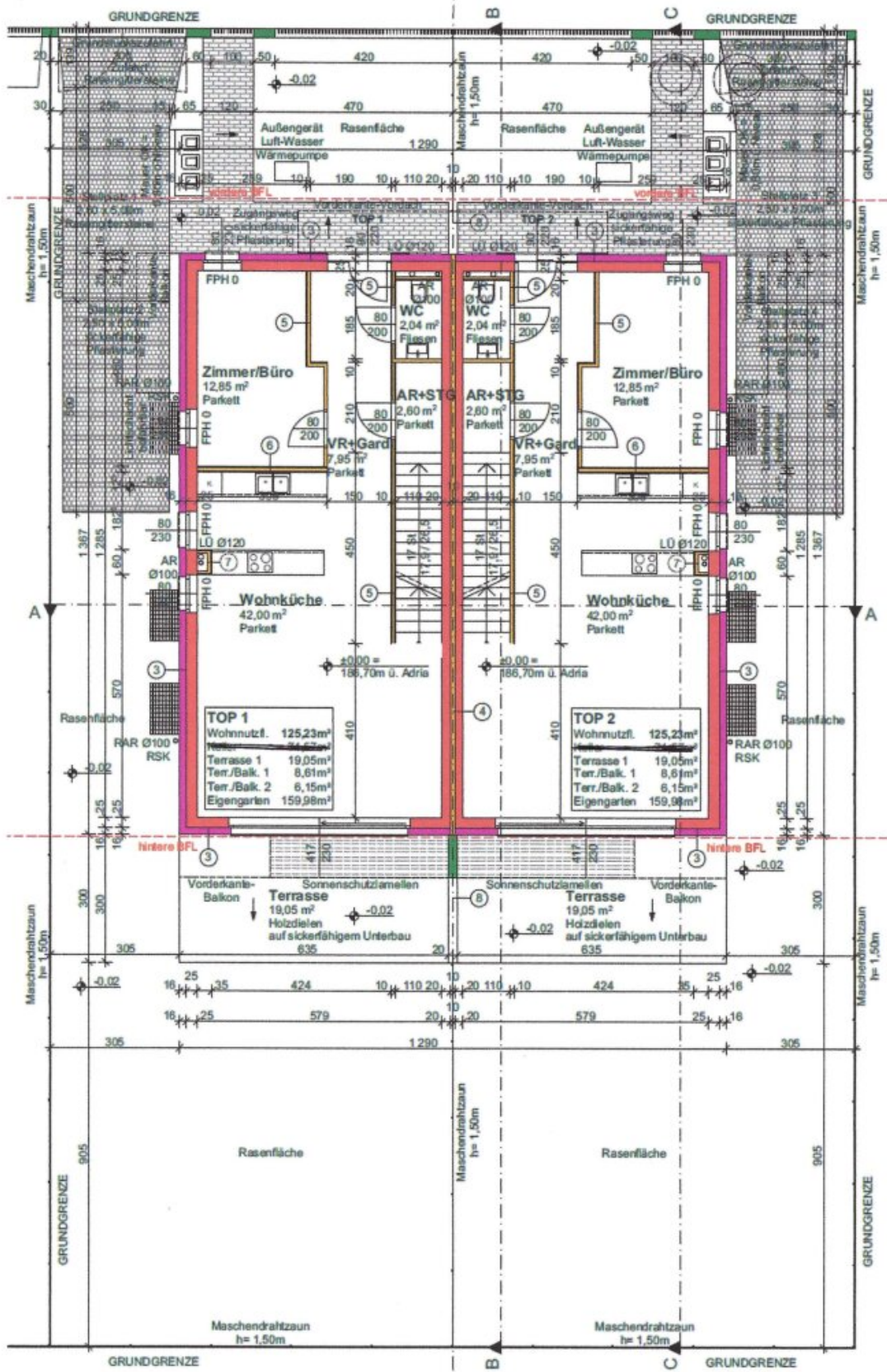
Erdgeschoß M1:100
