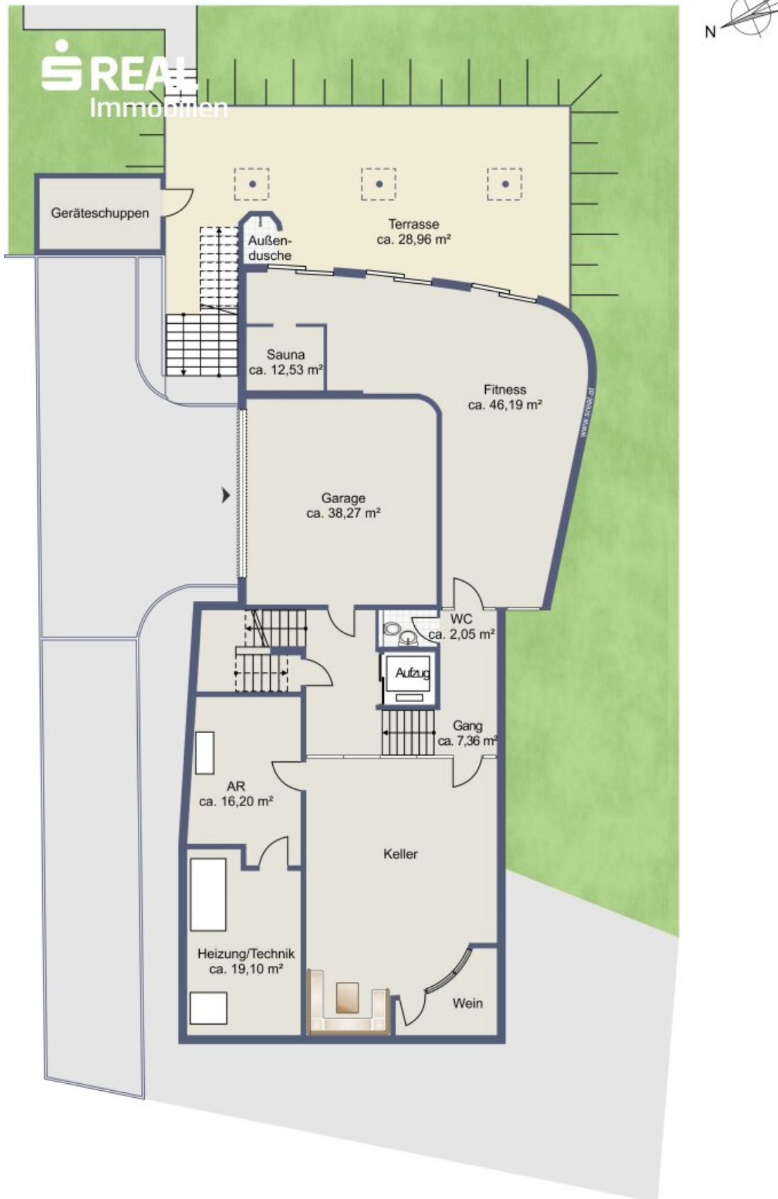
Skizze Kellergeschoss
