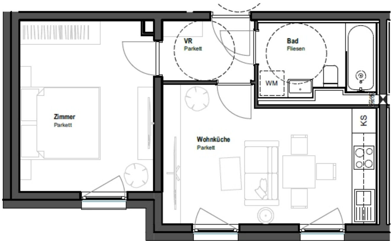
Grundriss 1:50
