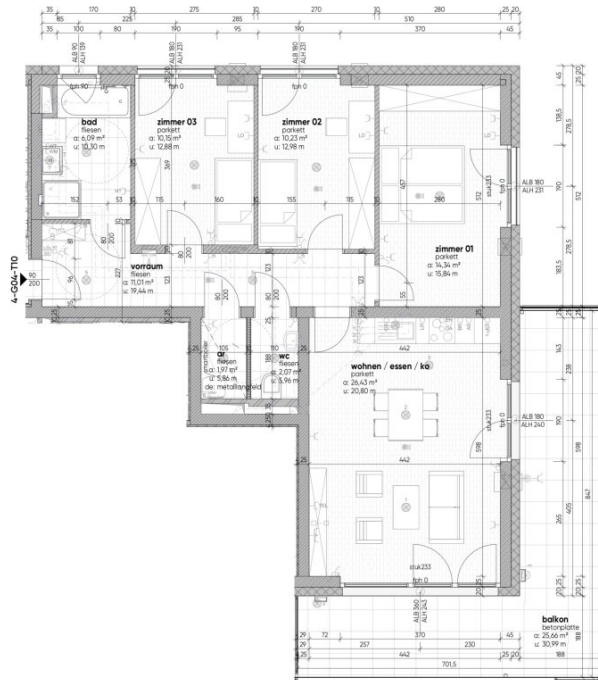
grundriss mit technik M1:75
