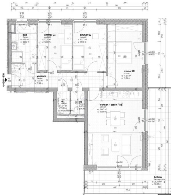
grundriss mit techn M1:75
