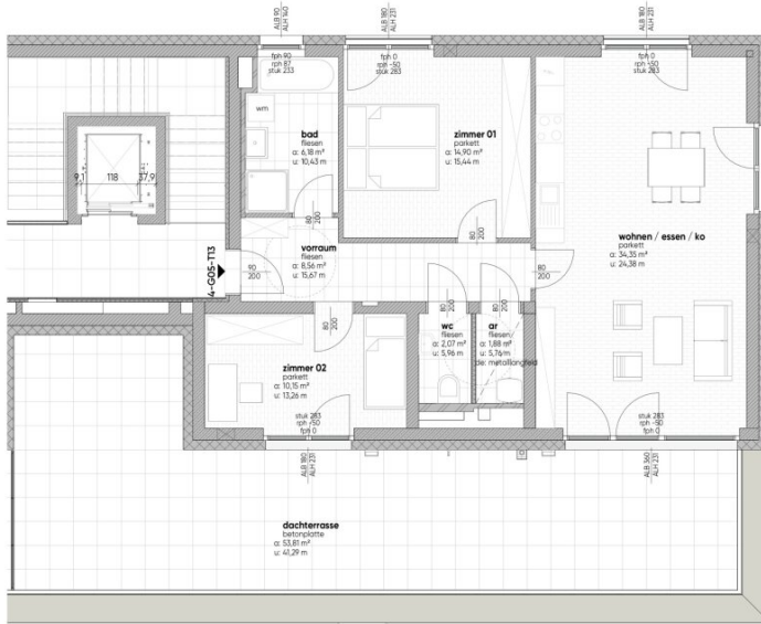
grundriss M1:75
