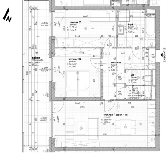
grundriss mit technik M 1:75
