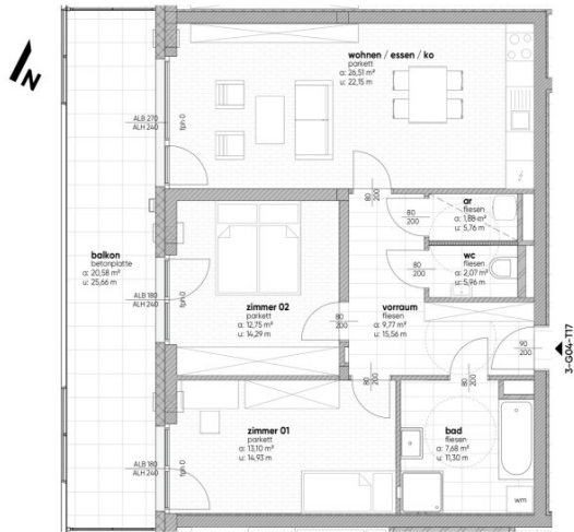
grundriss M 1:75
