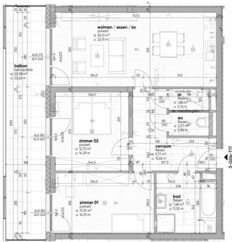
grundriss mit technik M 1:75
