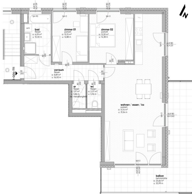
grundriss M1:75
