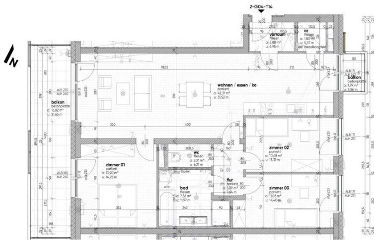
grundriss mit technick N1:75
