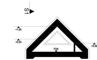
Schnitt 2
