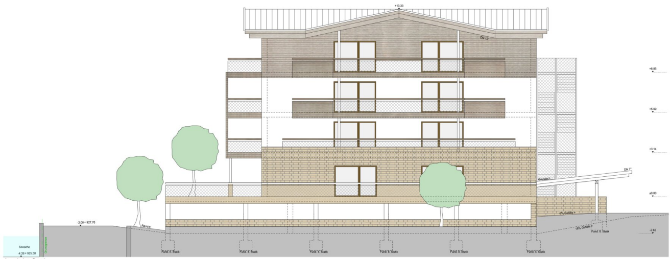
Ansicht Süd
