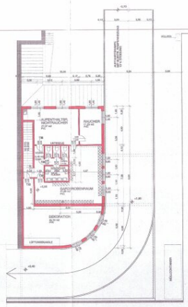
1. OBERGESCHOSS
