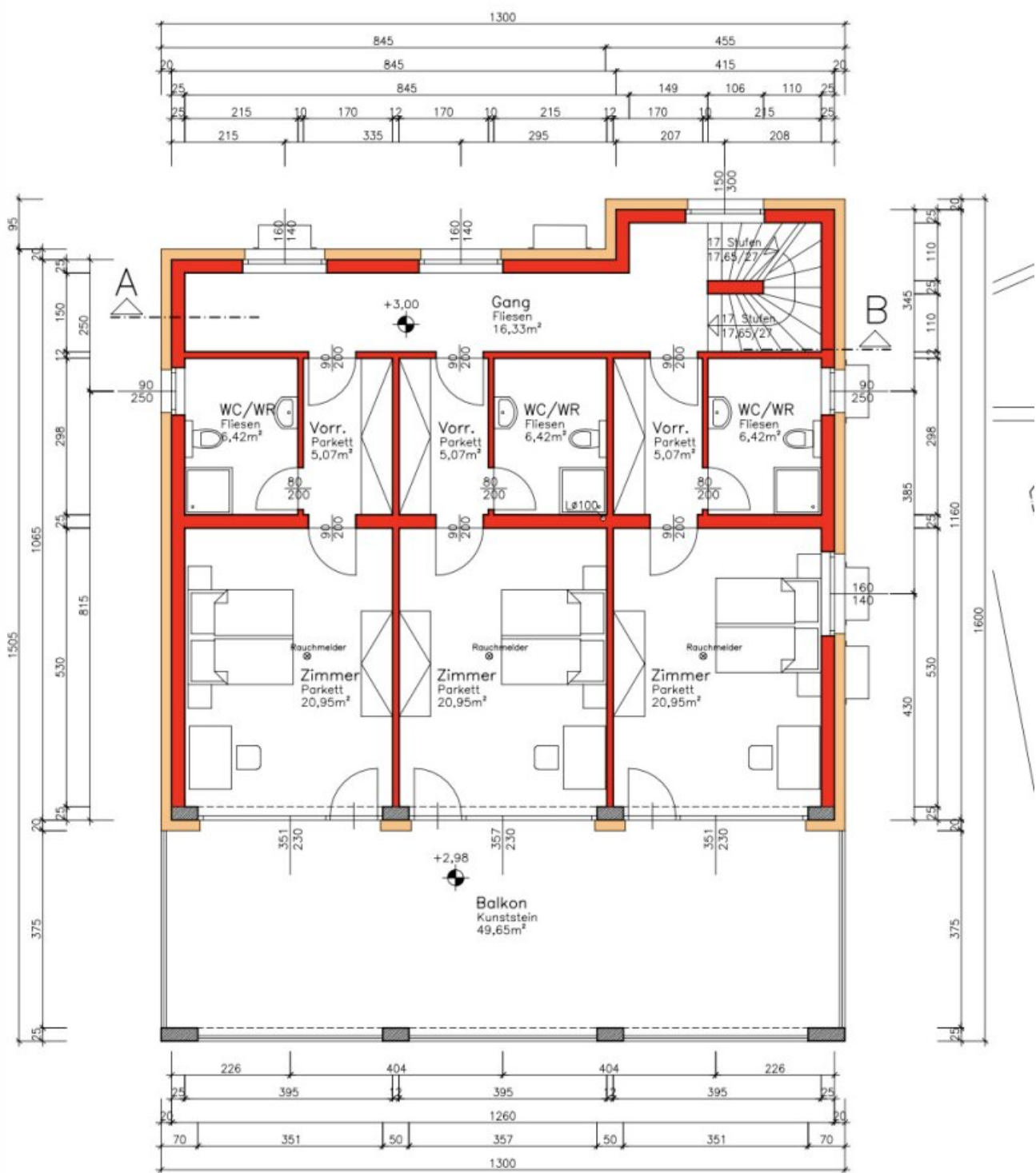
Obergeschoß 113,65m 2
