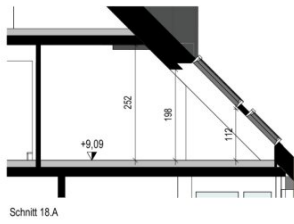
Schnitt 18.A
