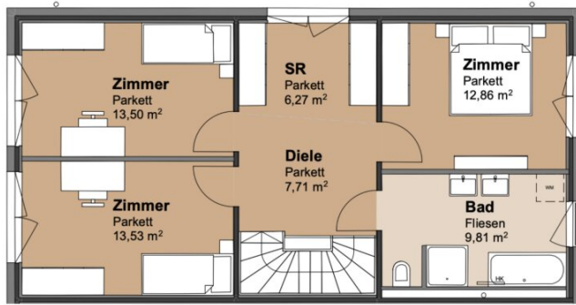
Obergeschoss
