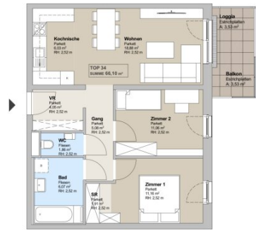
2. Obergeschoß M: 1: 100
