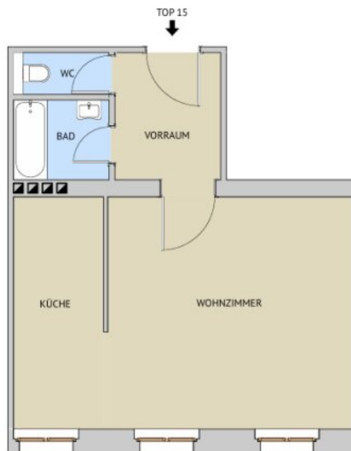
GRUNDRISS M 1:100
