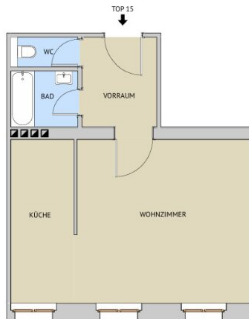
GRUNDRISS M 1:100
