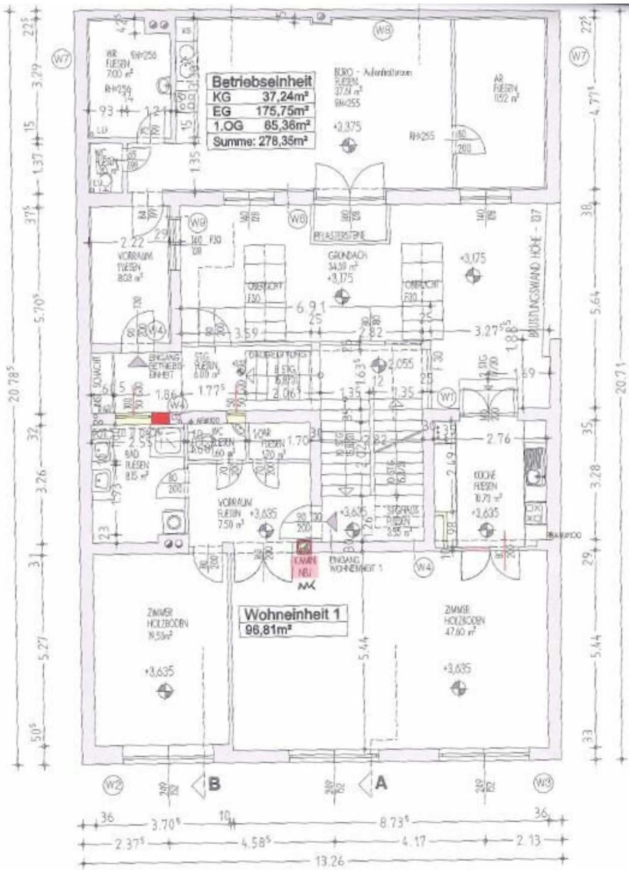
1. OBERGESCHOSS
