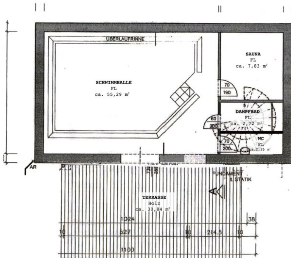
2. UNTERGESCHOSS
