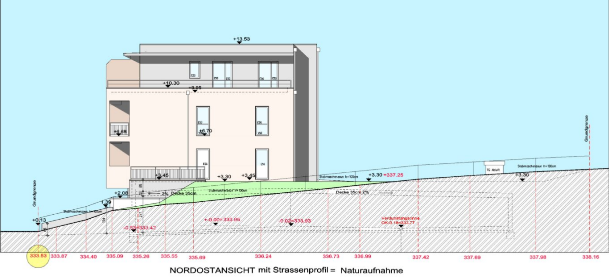
NORDOSTANSICHT mit Strassenprofil = Naturaufnahme
