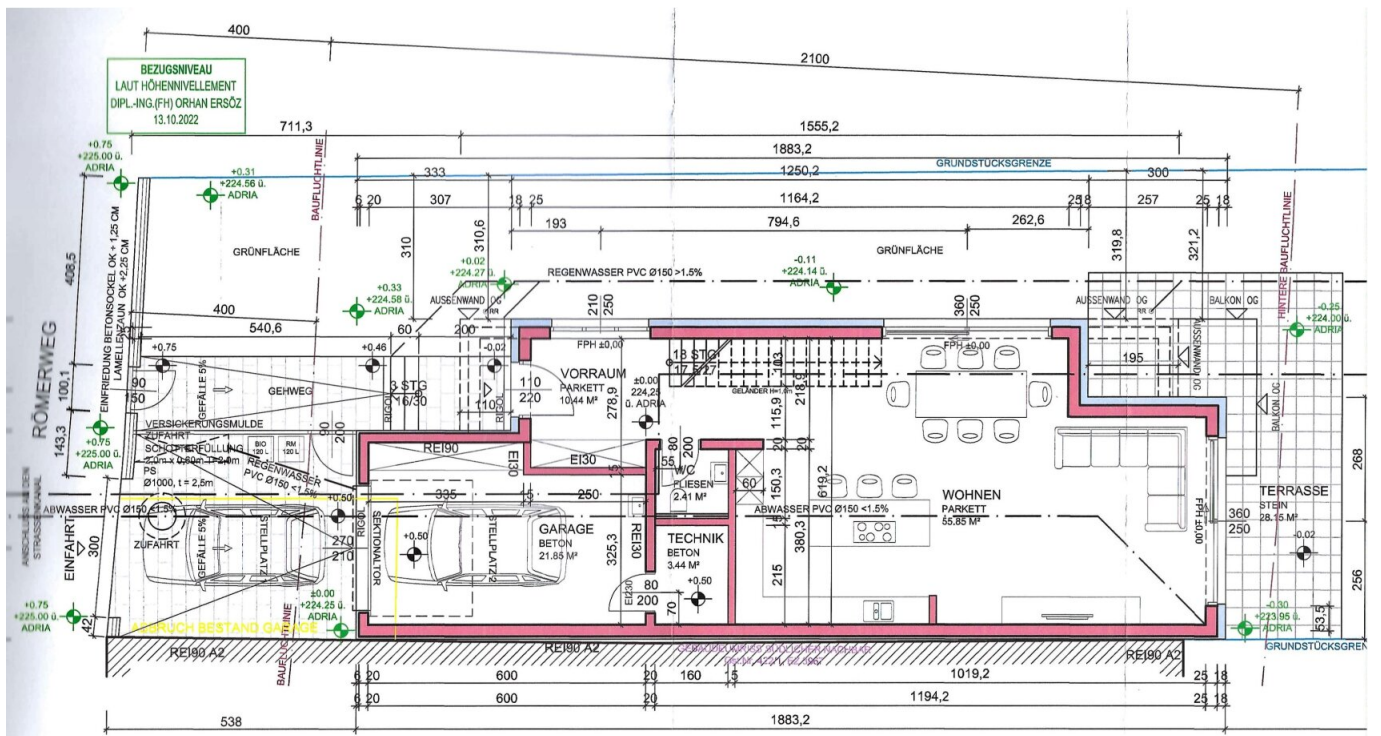
ERDGESCHOSS M 1:100
