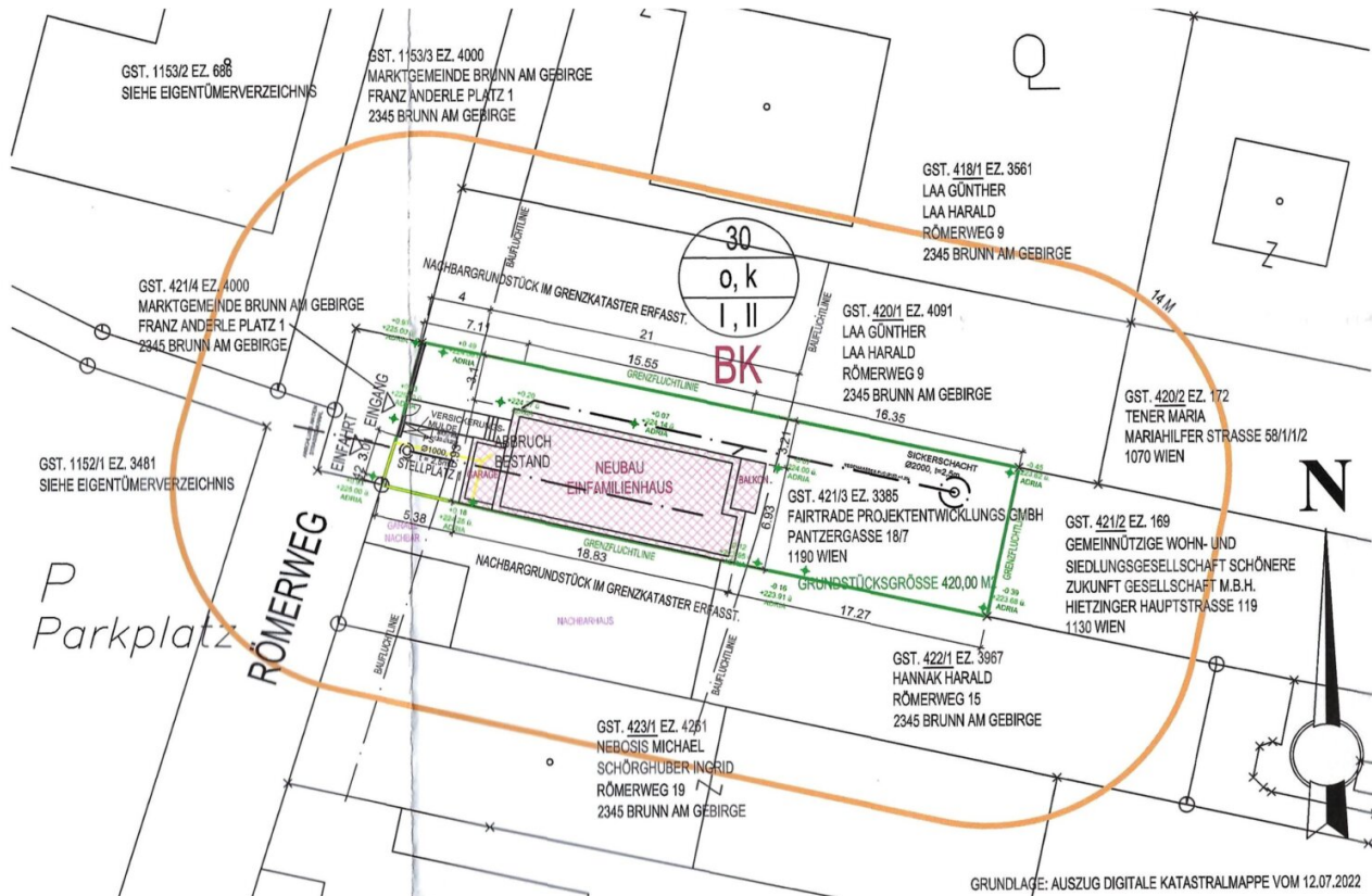
LAGEPLAN M 1:500
