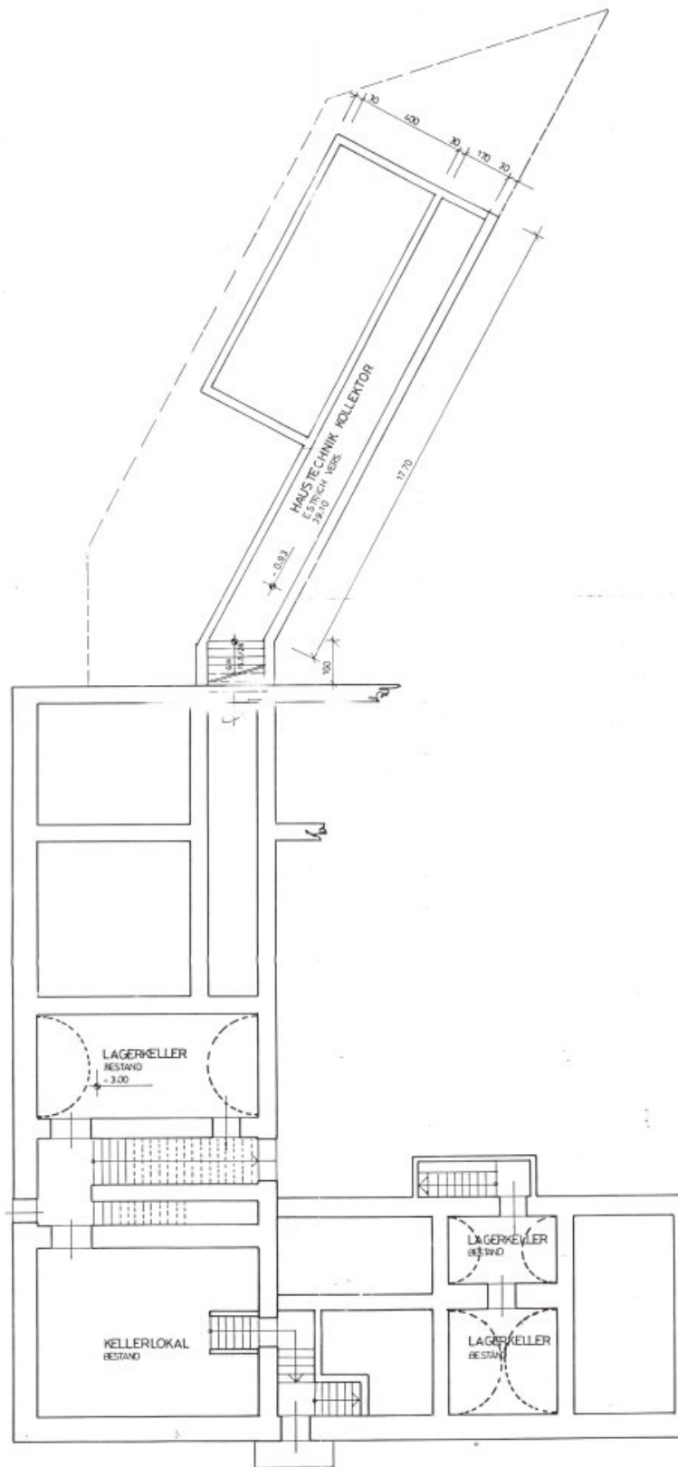
GRUNDRISS KELLERGEHOSS
