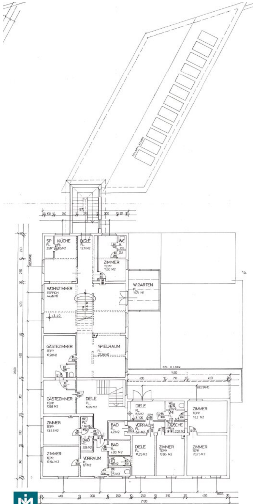
GRUNDRISS 1. OBERGESCHOSS
