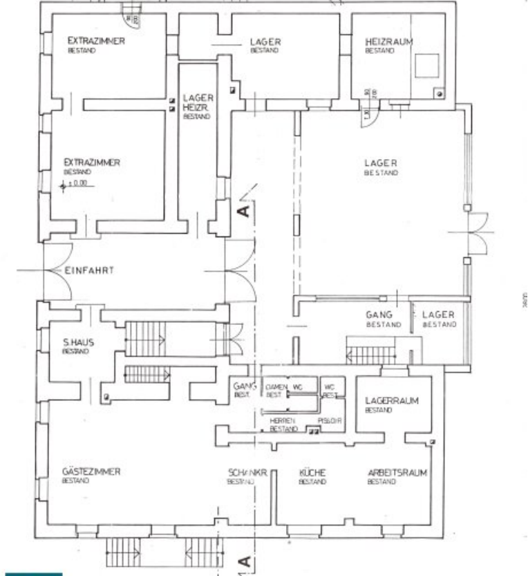
M NDRISS ERDGESCHOSS KANAL BESTAND
