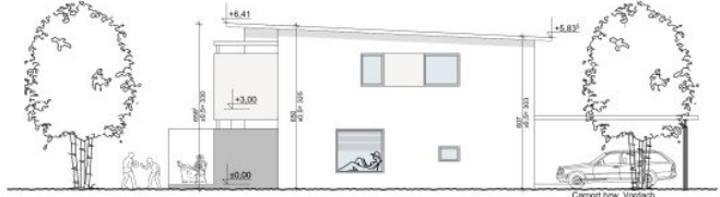
Nord-Ostansicht
