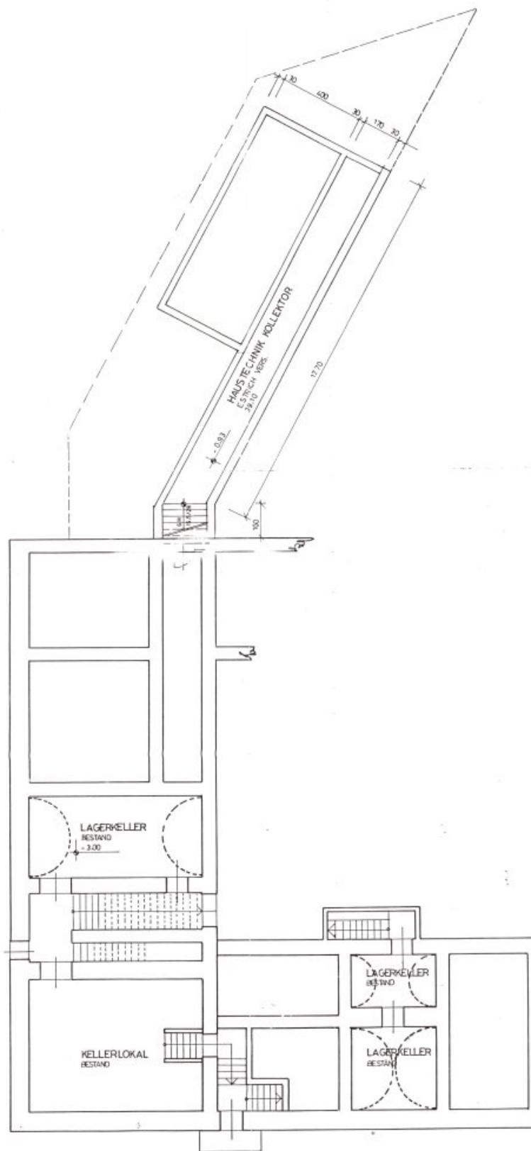
GRUNDRISS KELLERGESCHOSS
