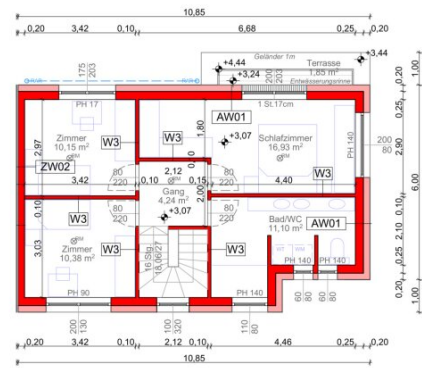
GRUNDRISS OBERGESCHOSS 1:100
