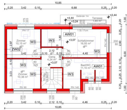
GRUNDRISS OBERGESCHOSS 1:100
