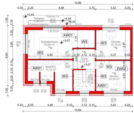
GRUNDRISS OBERGESCHOSS 1:100
