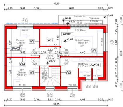
GRUNDRISS OBERGESCHOSS 1:100
