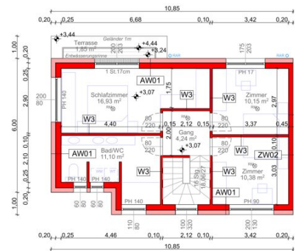
GRUNDRISS OBERGESCHOSS 1:100
