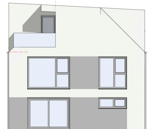
A1 Ansicht SÜD 1:100
