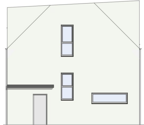
A4 Ansicht NORD 1:100
