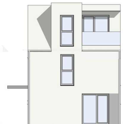
A1.1 Ansicht WEST 1:100
