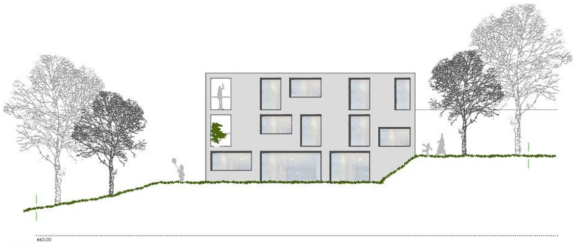
ansicht ost haus b
