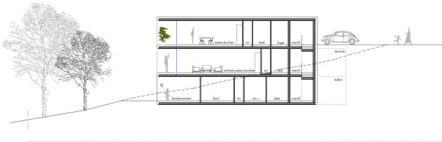
schnitt s1 - s1
