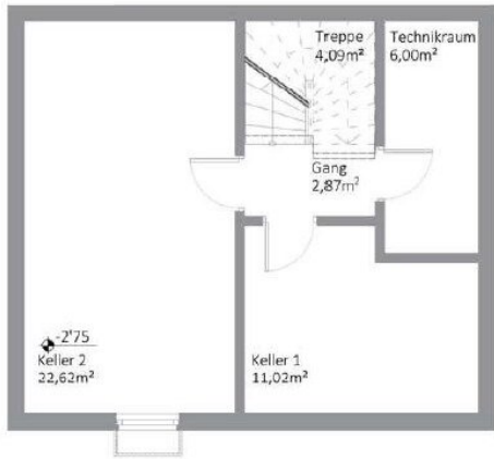
KELLERGECHOSS NF 46,60m 2
