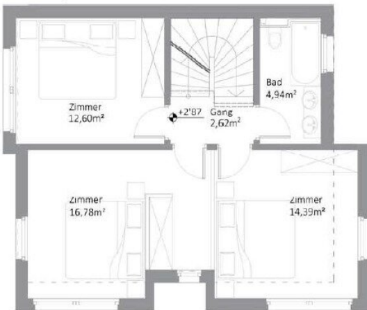
OBERGECHOSS WNF 51,33m 2
