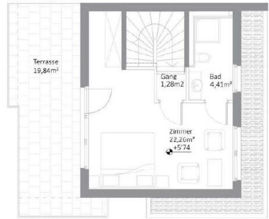
DACHGESCHOSS WNF 27,95m 2
